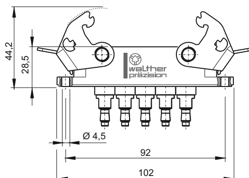
Festhälfte / fixed half 90410-4-...
