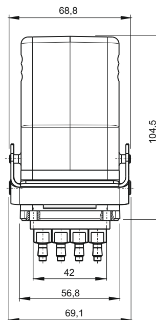
gekuppelter Zustand connected condition
